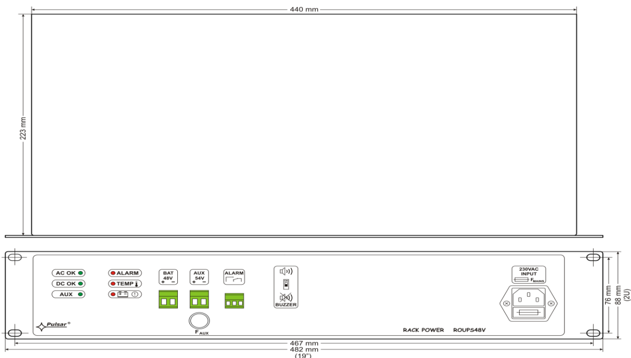
Rys.3. Widok zasilacza.
